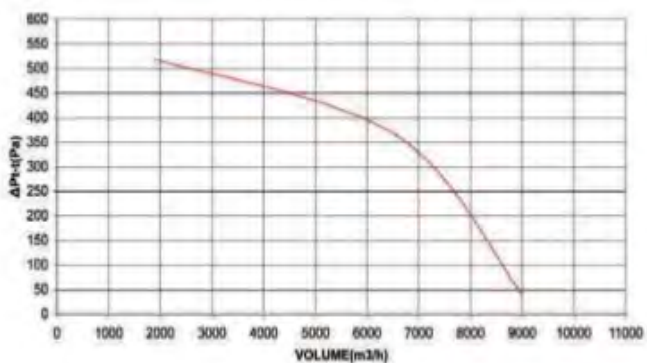
Φ350-5.5HP-1450RPM
