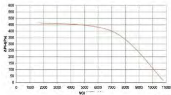
Φ450-5.5HP-950
