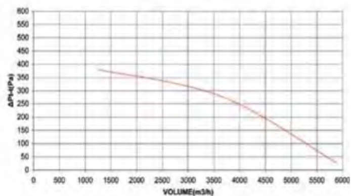
Φ350-2.0HP-950RPM
