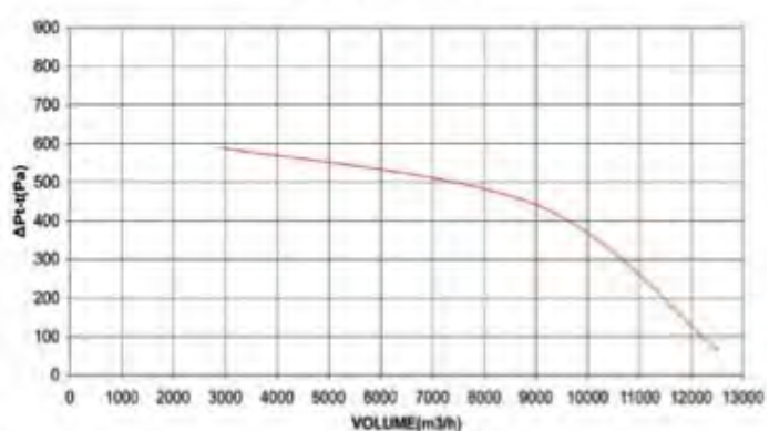
Φ450-4.0HP-950RPM
