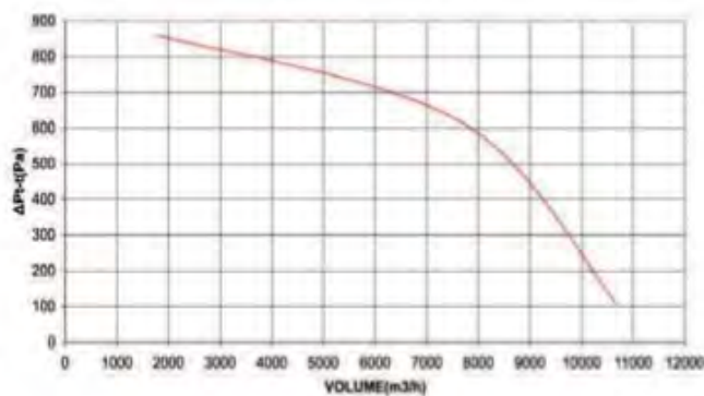
Φ450-7.5HP-1450RPM Φ500-10HP-1450RPM
