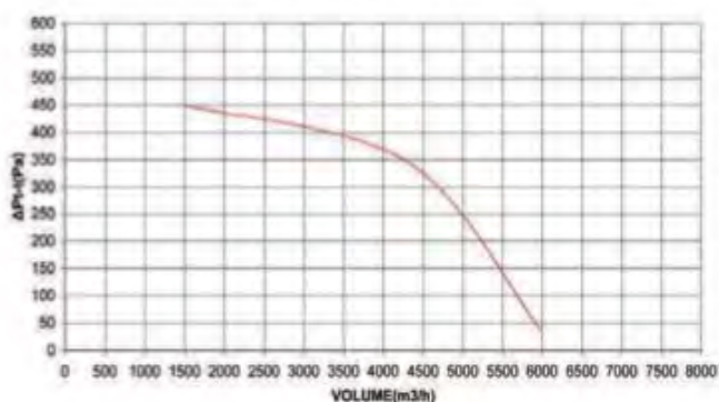
Φ250-1.5HP-1450RPM
