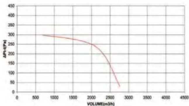
Φ200-0.5HP-1450RPM
