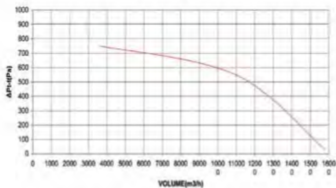
Φ450-5.5HP-950
