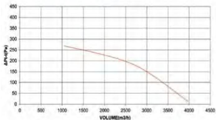
Φ350-1.5HP-950RPM
