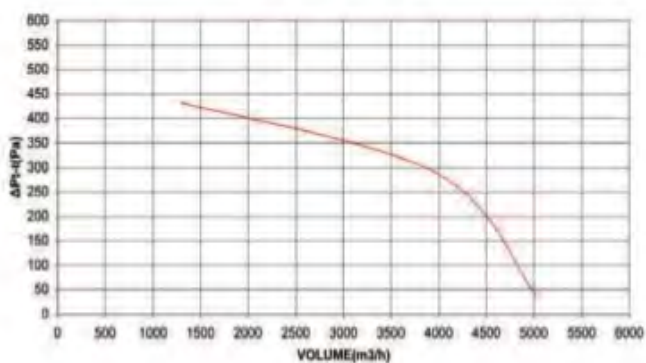
Φ250-1HP-1450RPM
