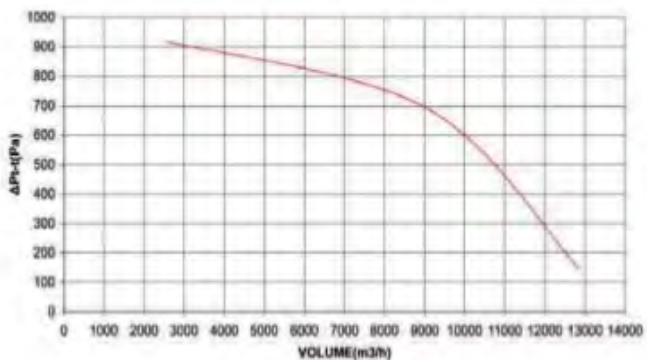
Φ350-5.5HP-1450RPM
