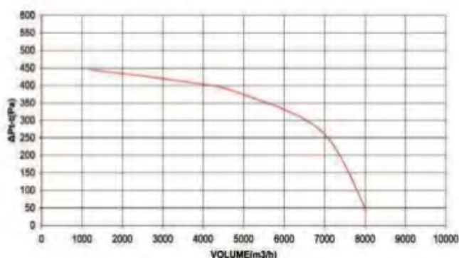
Φ300-2.0HP-1450RPM
