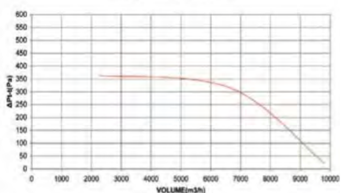
Φ450-4.0HP-950RPM
