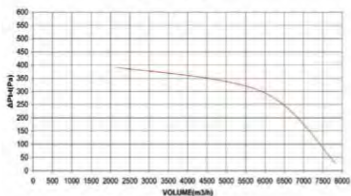
Φ350-3.0HP-950RPM
